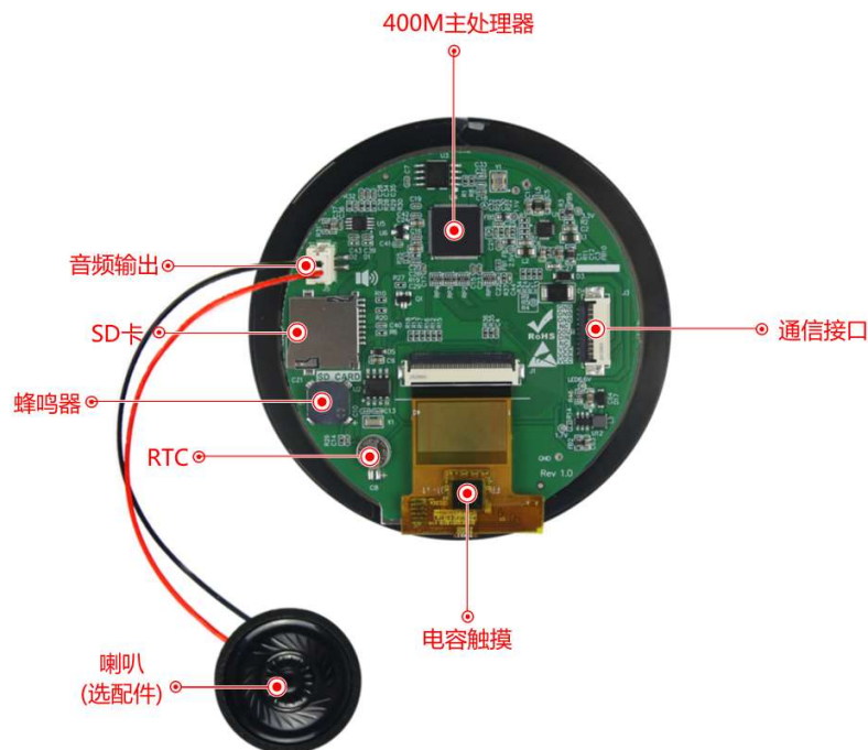
图 1-2 硬件配置图
